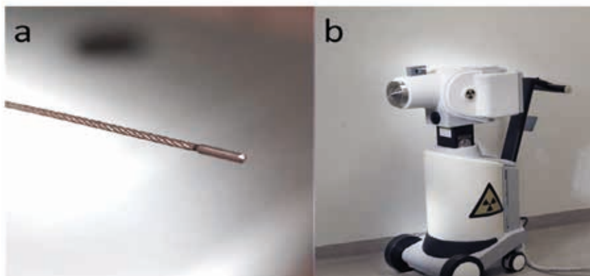
Fig. 1. (a) Visar en kapslad källa svetsad till en wire och (b) en behandlingsutrustning. MicroSelectron HDR (Elekta AB, Stockholm, Sverige)
